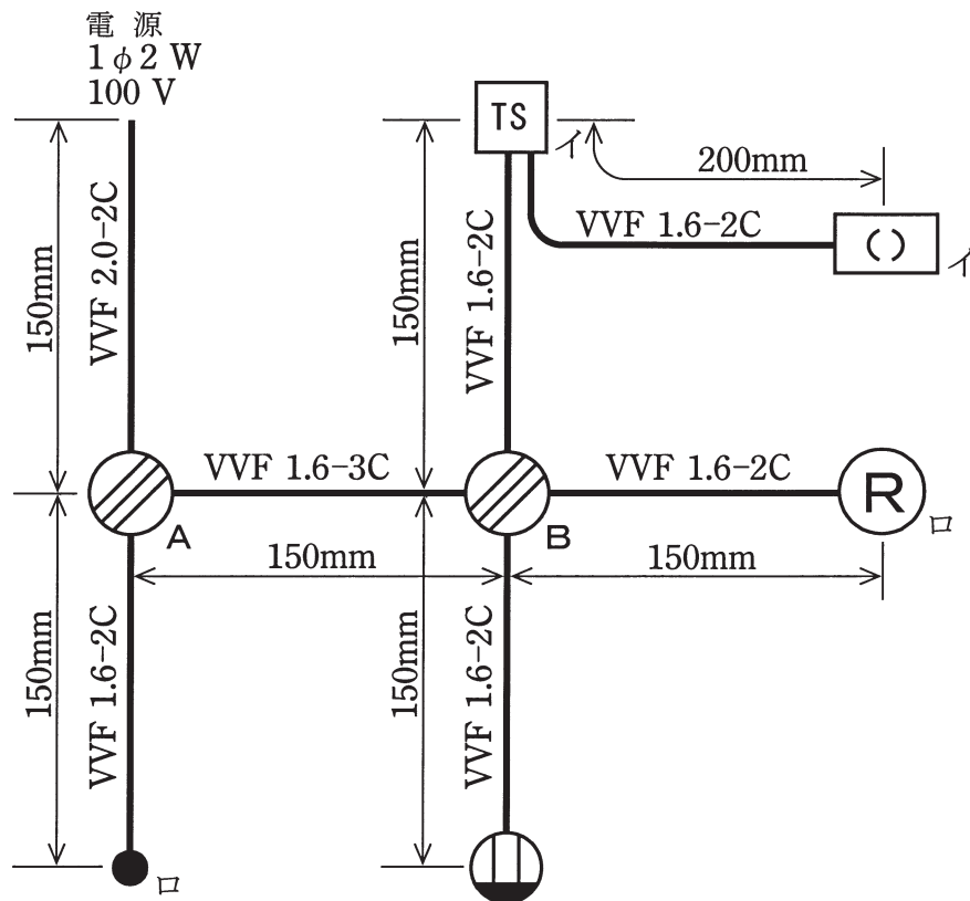
図 1. 配線図
