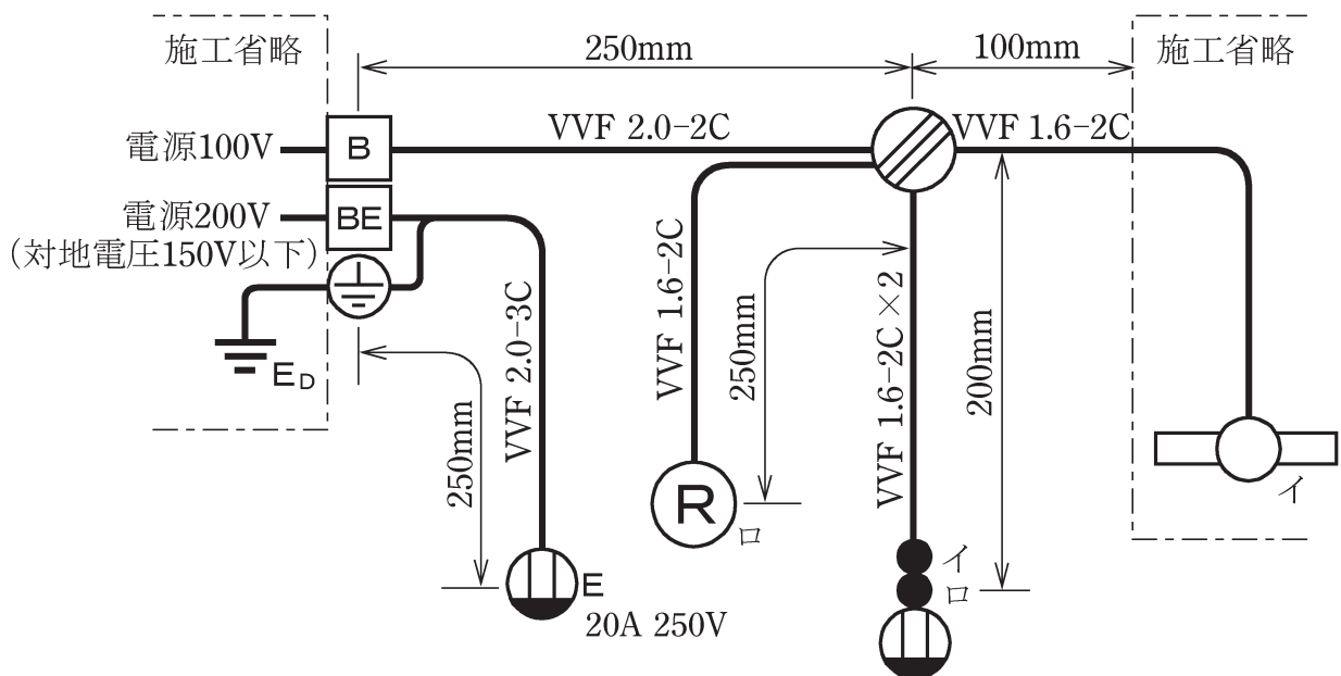
図 1. 配線図
